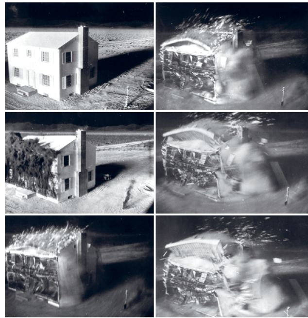
Bildeserie av et hus 1 km fra hyposenteret ved en atomprøvesprengning i Nevadaørkenen i 1953. Det går to sekunder mellom første og siste bilde.
